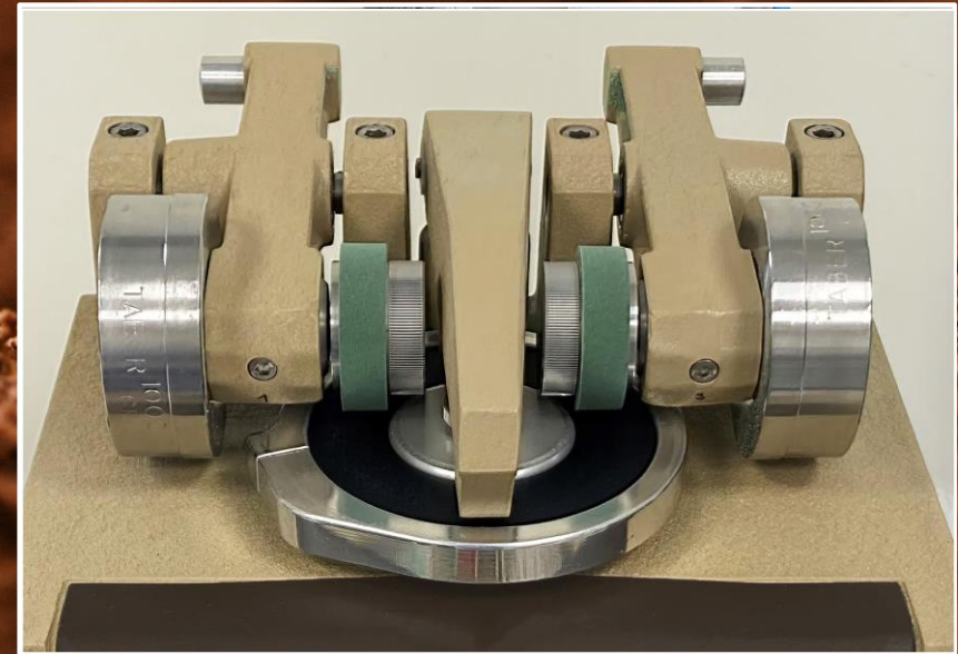
Teste de abrasão Taber®
