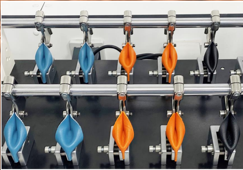
Teste de resistência à flexão
